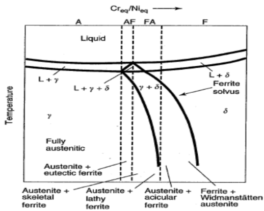
شکل 3- رابطه بین نوع انجماد و نمودار فاز شبه دوتایی [27].
